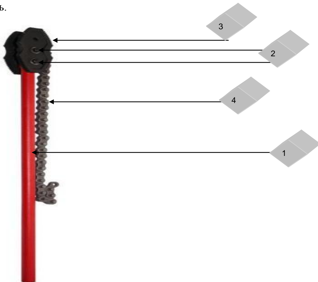
Рис 1. Устройство ключа. 1. Ручка. 2. Двухсторонние щетки. 3. Болты крепления щечек. 4. Цепь.
